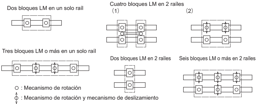
Fig.4 Ejemplos de mecanismos de mesas
