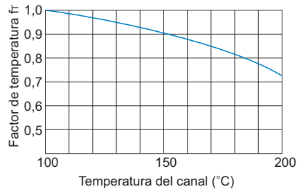
Fig.9 Factor de temperatura (f T )
