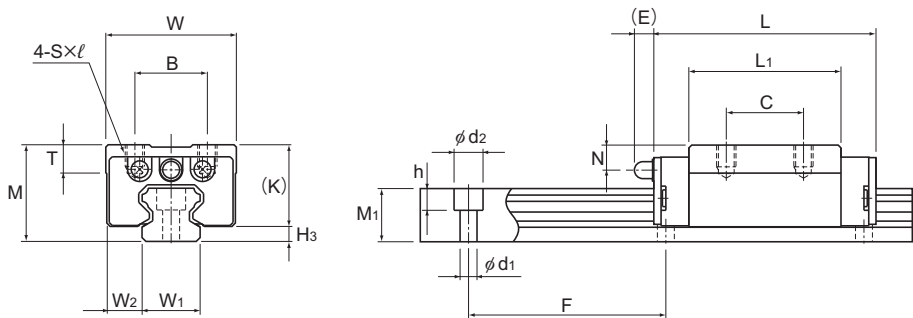
Modelo HSR12RM
