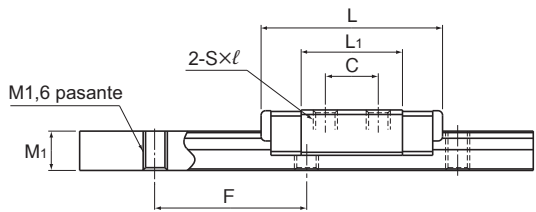
Modelo RSR3M
