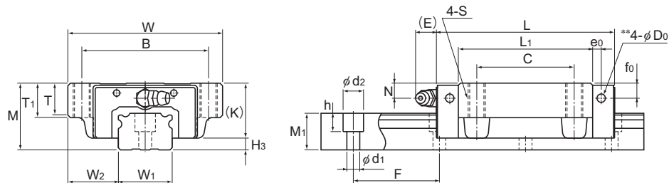
Modelo NRS-A
