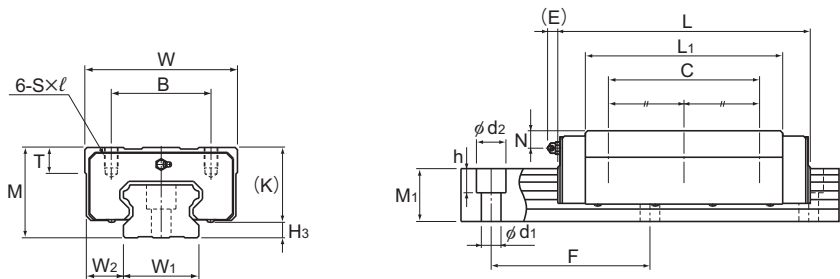
Modelos HSR100 a 150HR
