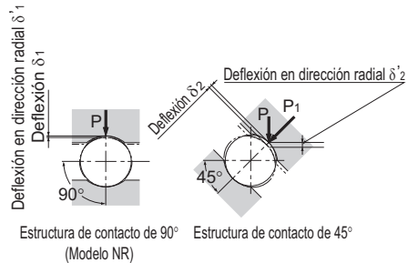
Fig.1 Deflexión bajo carga radial
