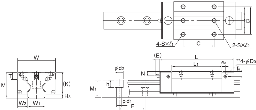
Modelos SRG15V y 20V/LV
