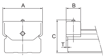
Fig.1 Pieza terminal EP para modelos NR/NRS
