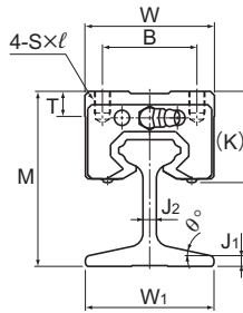
Modelo JR-R
