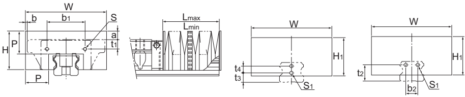
Modelos SHS15 a 30 Modelos SHS35 a 65 Unidad: mm
