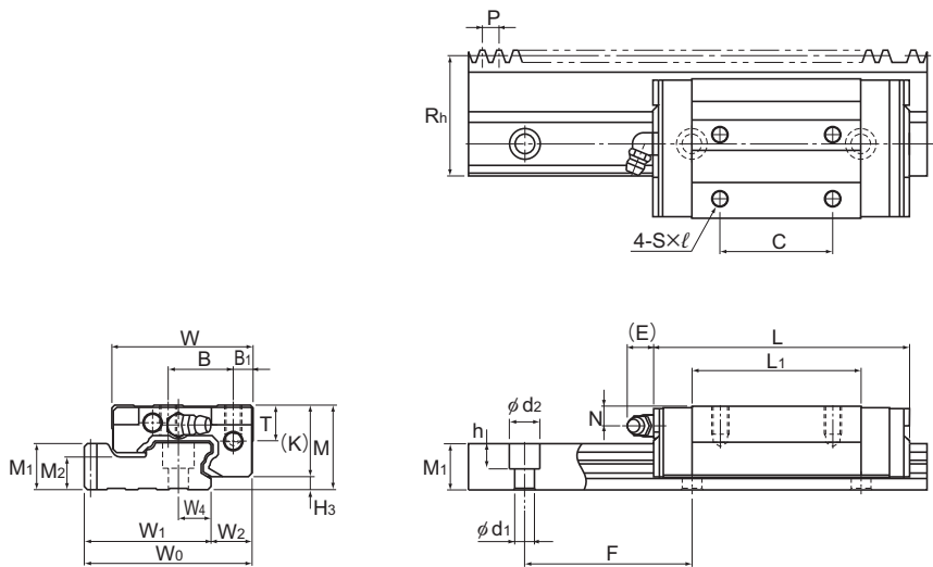
Modelo GSR-T-R
