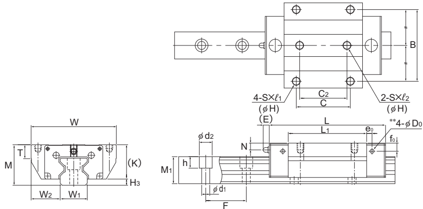
Modelos SRG15A y 20A/LA
