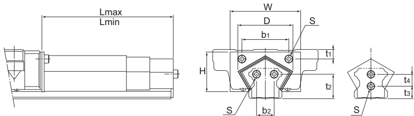
Modelos HSR25 y 30
