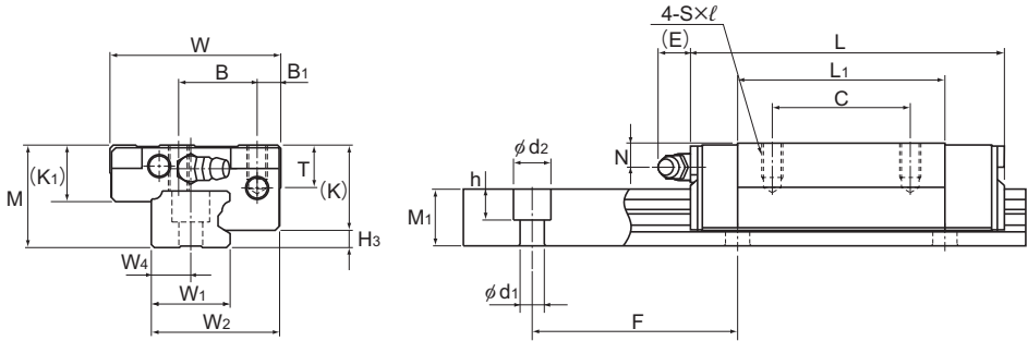
Modelos GSR20 a 35T, Modelos GSR20V y 25V
