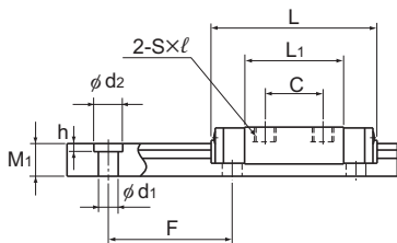
Modelo RSR5N
