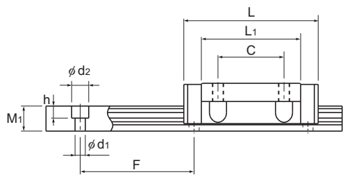
Modelos SHW17CAM y SHW21 a 50CA
