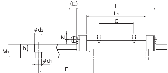
Modelos RSR15 y 20VM/N
