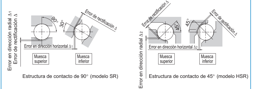
Fig.2 Error de mecanizado y precisión
