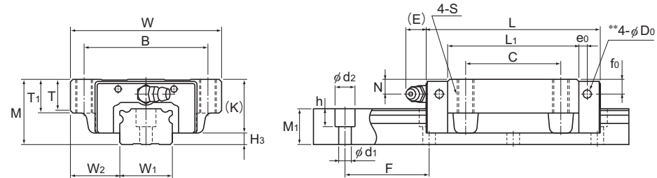
Modelo NR-A
