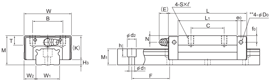
Modelo NR-R
