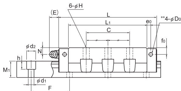
Modelo NR-LB
