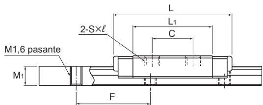
Modelo RSR3N
