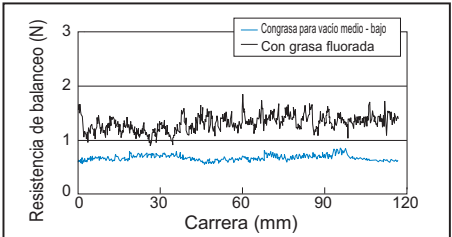
Fluctuación de la resistencia a la rodadura
