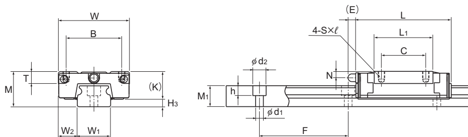
Modelo RSR15ZM
