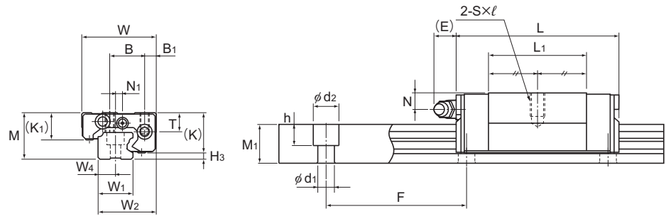
Modelo GSR15T/V
