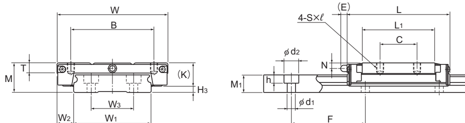
Modelo RSR15WZM
