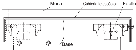
Fig.2 Ejemplo de montaje de fuelle
