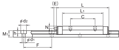
Modelo RSR14WVM
