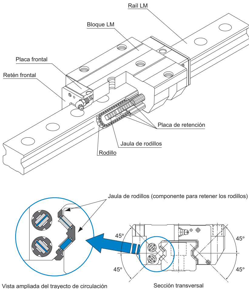
Fig.1 Plano estructural del modelo SRG de guía LM con jaula de rodillos
