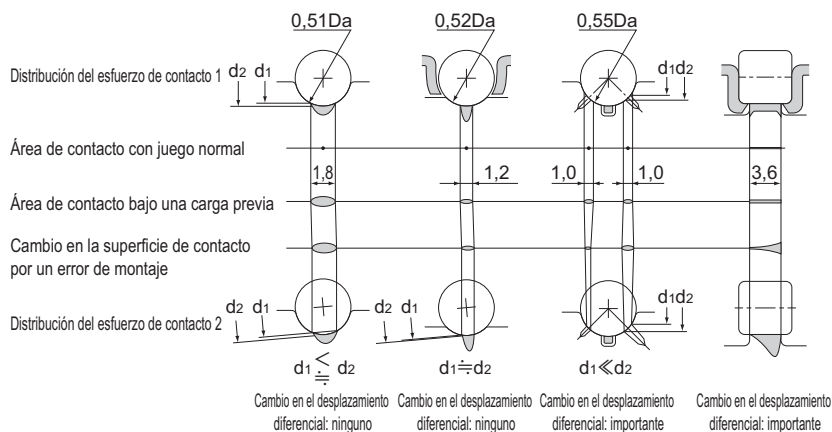
Fig.4 Comparación de la superficie de contacto ( \phi 6,350 bola, \phi 6 \times 6l rodillo)
