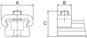
Fig.1 Tapón del modelo RSR-Z/RSR-WZ (tipo C)
