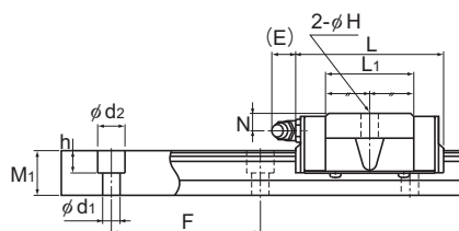
Modelo SR-SB
