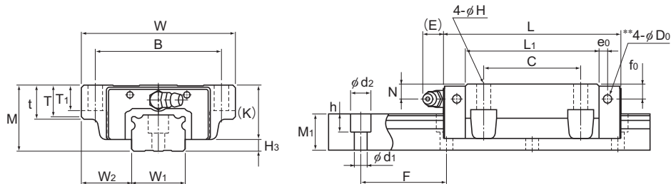
Modelo NR-B
