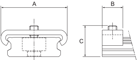
Fig.1 Tapón del modelo HRW (tipo C)
