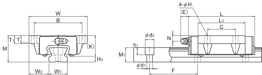
Modelo SR-M1TB
