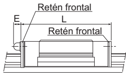
Fig.1 Dimensiones del engrasador para el modelo SRS
