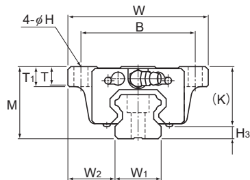
Modelos HSR20M1B/M1LB
