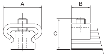
Fig.1 Tapón del modelo HSR (tipo C)
