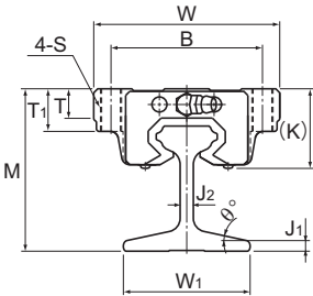
Modelos JR25 y 35-A
