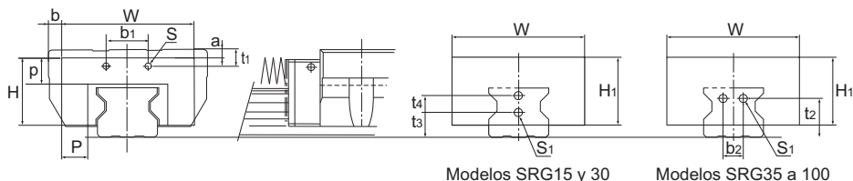
Modelos SRG15 y 30
