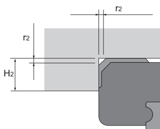
Reborde para el bloque LM
