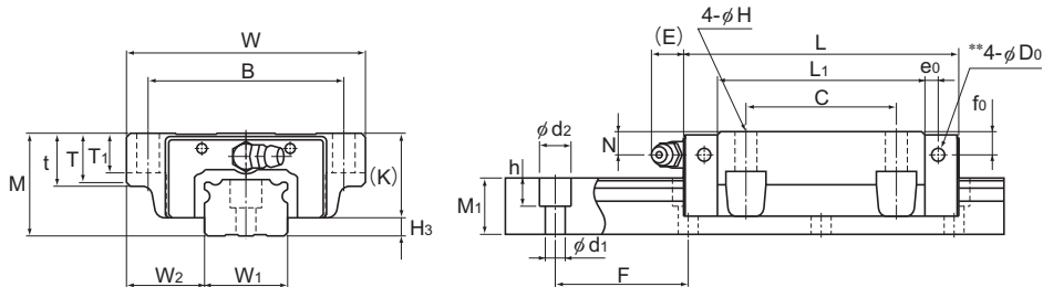
Modelo NRS-B
