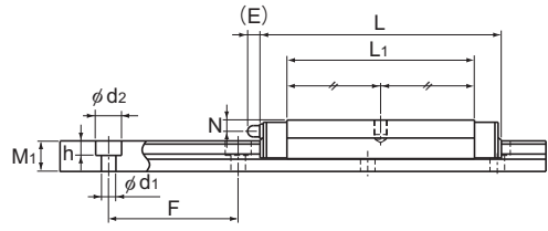
Modelos RSR5WTM/WTN
