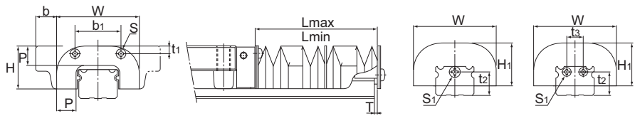
Modelos NR/NRS 25X a 45 Modelos NR/NRS 55 a 100
