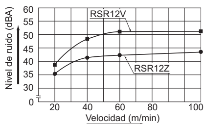
Fig.1 Niveles de ruido de los modelos RSR12Z y RSR12V
