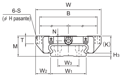
Modelos SHW17CAM y SHW21 a 50CA
