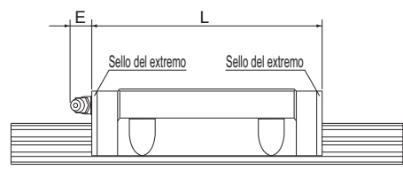
Fig.1 Dimensiones del engrasador para el modelo SHW
