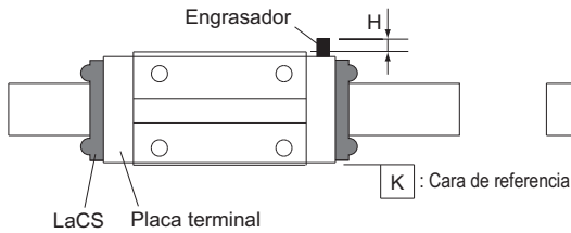
Ubicación de montaje del engrasador para los modelos SHS, SSR, SVR/SVS, SRG y NR/NRS
