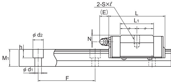
Modelo SR-M1V
