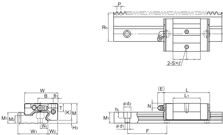
Modelo GSR25V-R
