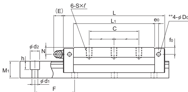
Modelo NR-LR
