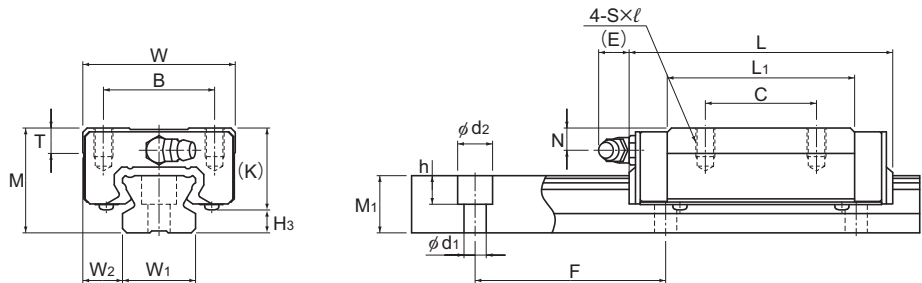
Modelo SR-M1W
