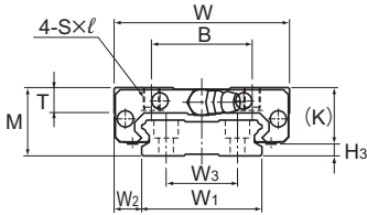
Modelos HRW17 y 21CR/CRM
