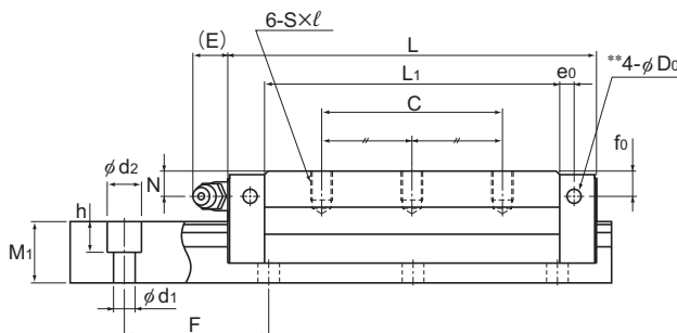
Modelo NRS-LR
