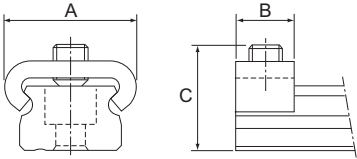
Fig.1 Tapón del modelo RSR-M1/RSR-M1W (tipo C)
