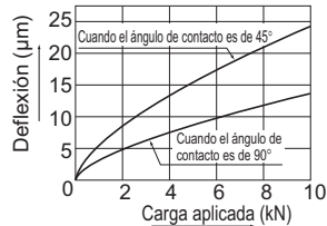
Fig.2 Carga radial y deflexión (juego normal, sin carga previa)
