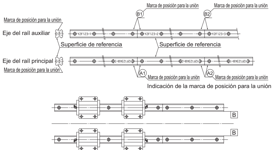
Fig.23 Uso de raíles empalmados
