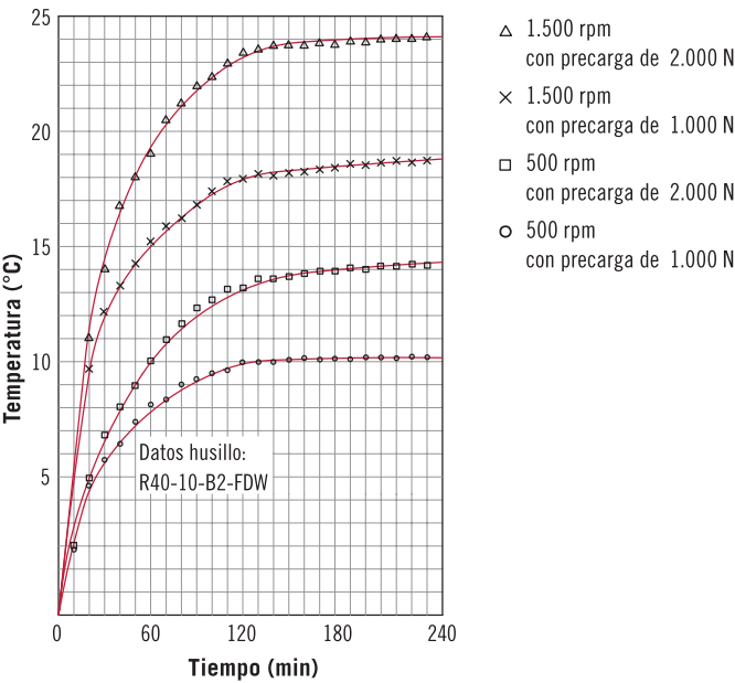
Fig. 3.26 Relación entre velocidad de funcionamiento, precarga y aumento de temperatura
