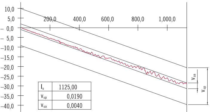
Fig. 3.14 Fluctuación de desplazamiento sobre trayectoria útil l_u
