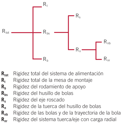
Fig. 3.25 Factores de rigidez para sistemas de alimentación con husillos de bolas
