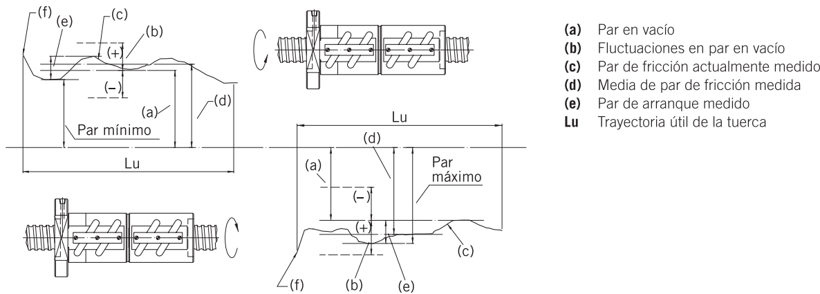
Fig. 3.19 Nomenclatura para pares en vacío medidos
