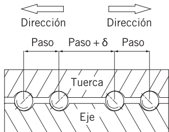
Fig. 3.17 Precarga por compensación del paso
