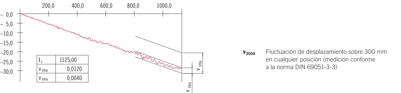
Fig. 3.12 Fluctuación de desplazamiento sobre trayectoria útil de 300 mm
