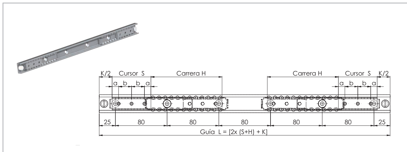
* Para los sistemas de las versiones 2 en el tamaño 63 con dos cursores independientes, la dimensión K cambia de 80 mm a 110 mm y para cada cursor adicional aumentar otros 30 mm.
