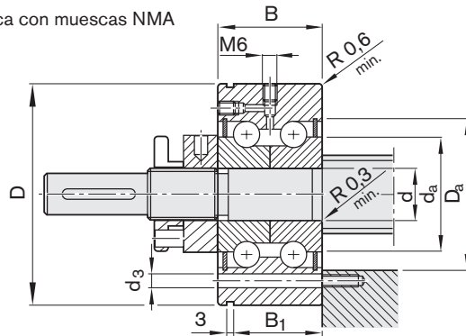
LGF-C-... con tuerca con muesca NMA
