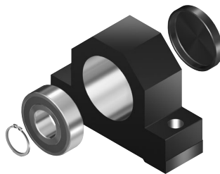
Módulo de grupo de componentes del soporte SEB-L
