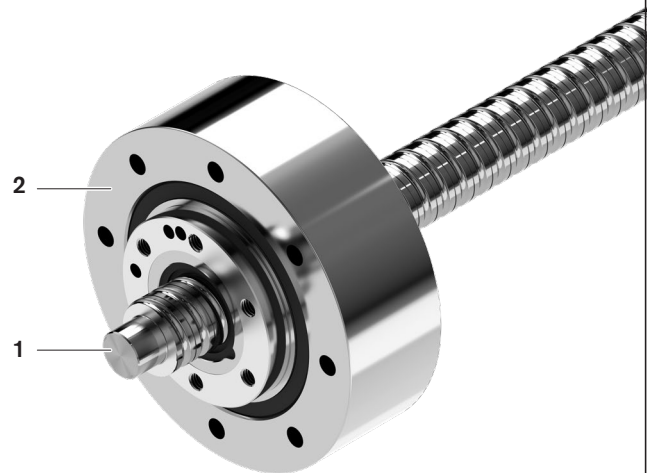
1 Husillo de husillo de bolas (BASA) 2 Tuerca accionada FAR
