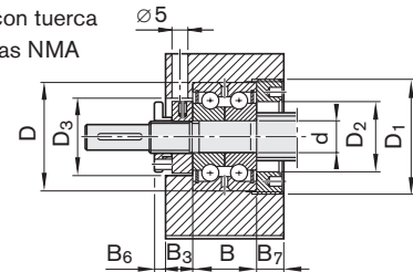
LGN-C...con tuerca con muescas NMA
