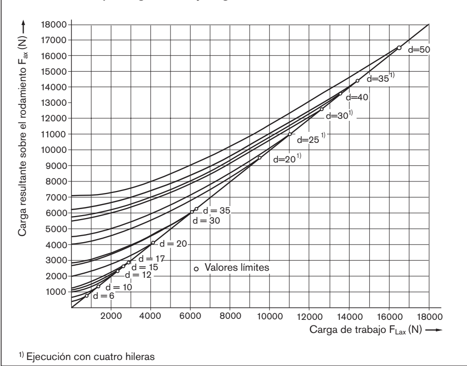
Valor límite de la precarga interna y carga resultante
